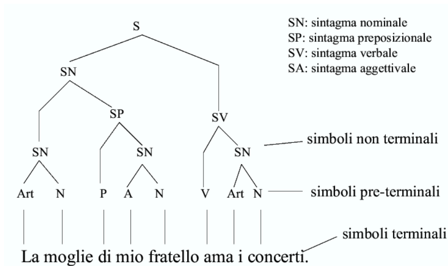
Figura 3.1: Albero sintattico
